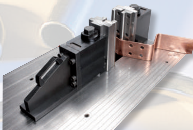
BUS BARS bending Îndoire de șuruburi U
